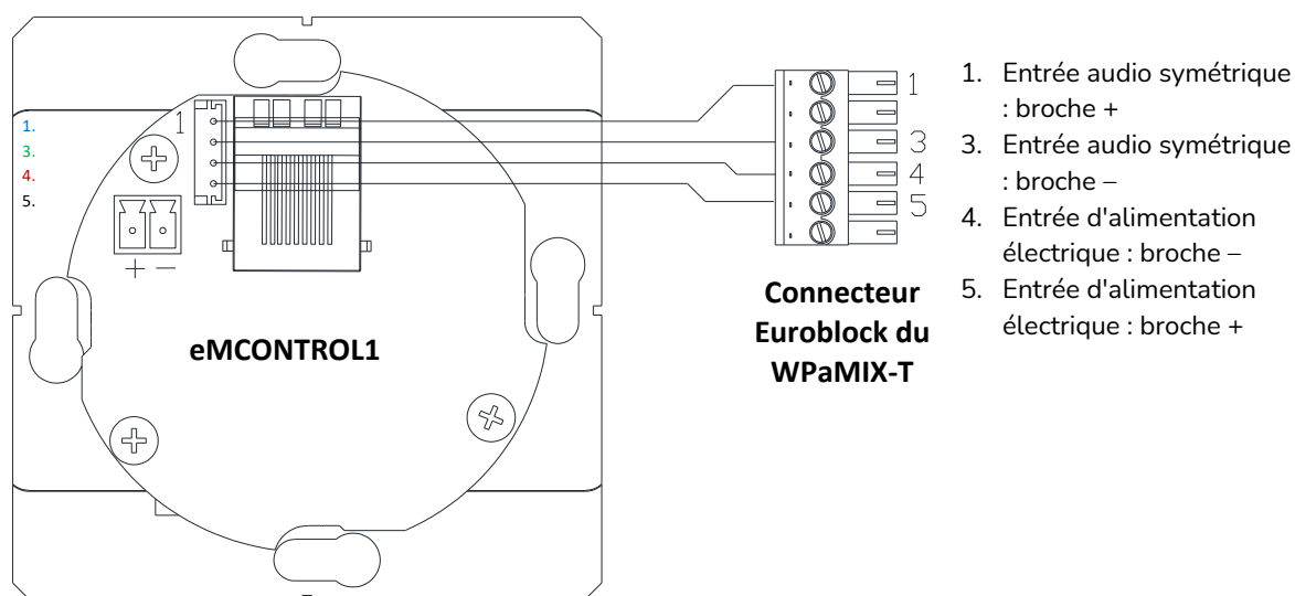
Figure 1 : schéma de raccordement eMCONTROL1 + WPaMIX-T
