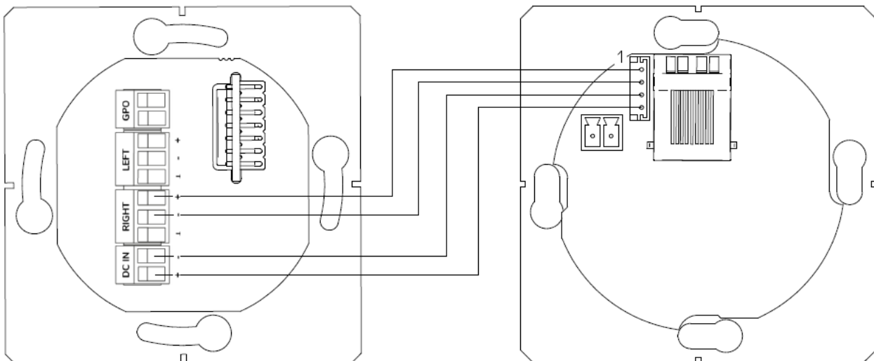
Abbildung 2 : Anschlussdiagramm WPaBT + eMCONTROL1
