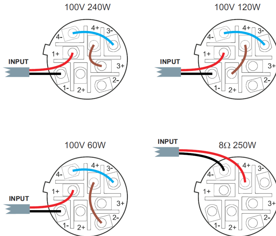
Abbildung 1: Anschlussdiagramm SpeakON®
