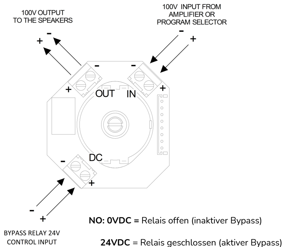
Abbildung 12: Anschlussdiagramm WPaH-AT6, WPaH-AT40 und WPaH-AT100
