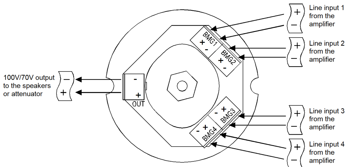
Abbildung 14: Anschlussdiagramm WPaH-SL4
