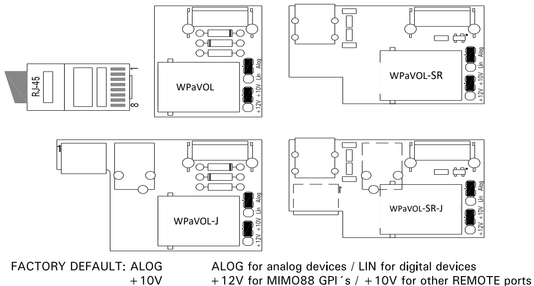
Abbildung 5: Interne Jumper
