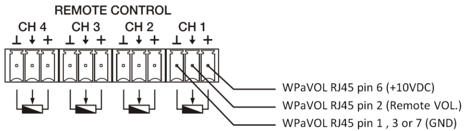
Abbildung 6: Anschluss WPaVOL / WPaVOL-SR an Fernbedienungs-Ports
