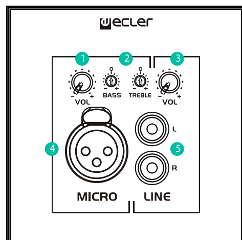
Abbildung 16: Funktionsdiagramm WPaMIX-T
